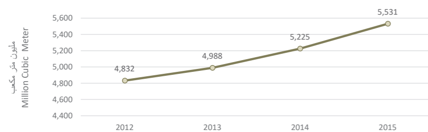
شكل 36: إنتاج مياه التحلية في مجلس التعاون 2012-2015م Figure 36: Desalinated Production in GCC 2012-2015
