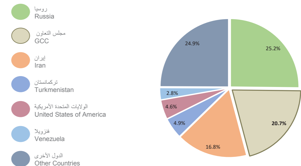
شكل 7: نسبة إنتاج الغاز الطبيعي في مجلس التعاون مقارنة ببقية الدول - 2016م Figure 7: Percentage of Natural Gas Reserves in GCC Compared to other Countries - 2016
