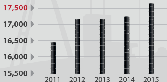
إنتاج النفط في مجلس التعاون الخليجي خلال الفترة 2011- 2015م
